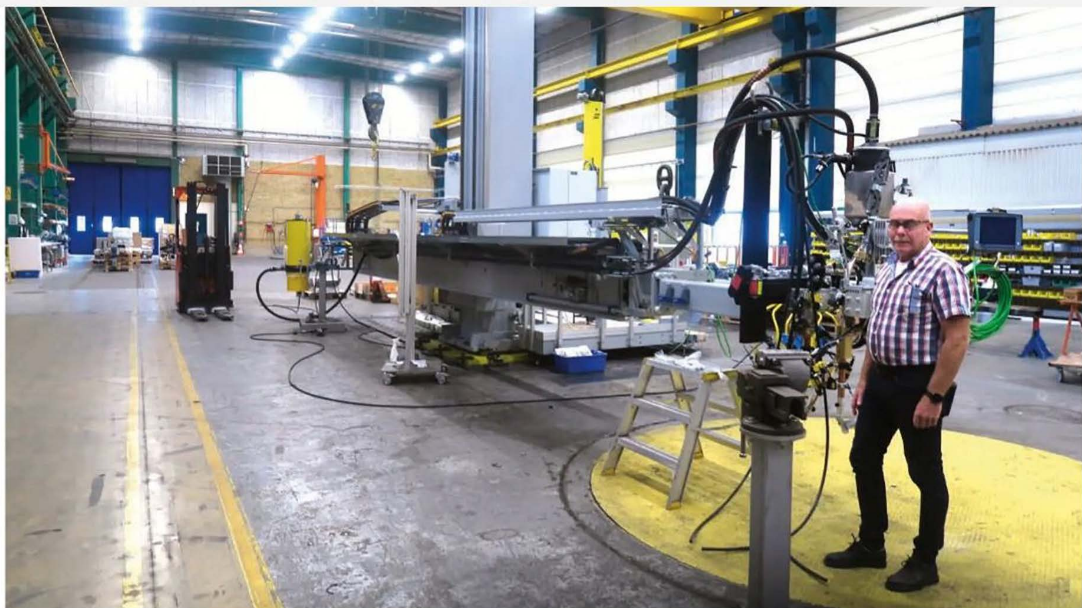
En specialsvets för vindkraftstorn med en cirka 12 meter lång teleskoparm håller på att monteras på Esab i Laxå. Den kan man få se på öppet hus på lördag, berättar Håkan Persson, jubileumsgeneral.
